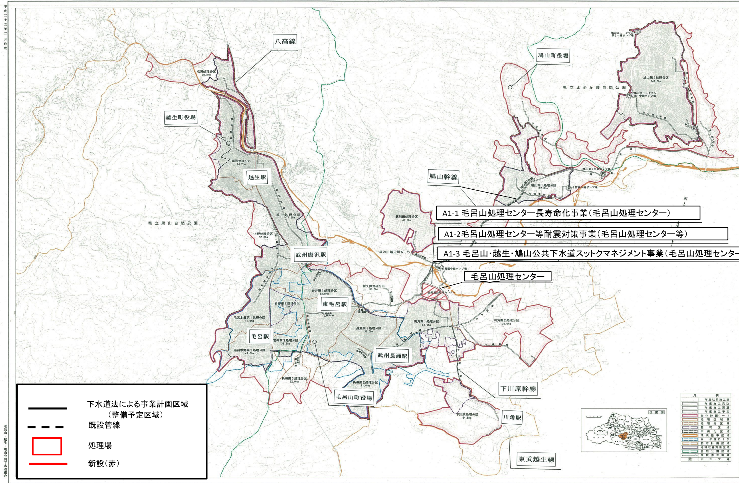
毛呂山・越生・鳩山公共下水道事業計画図 (污水)
